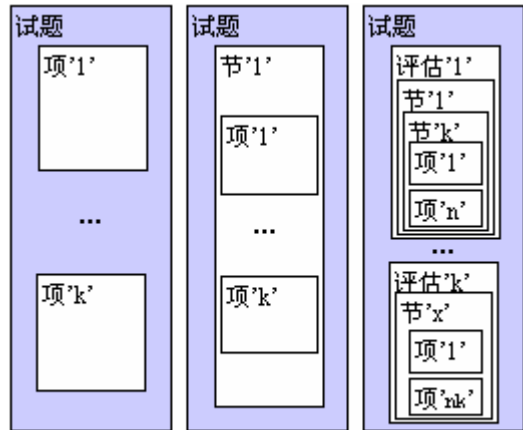
图 1.1 可互换的 QTI 核心数据结构
