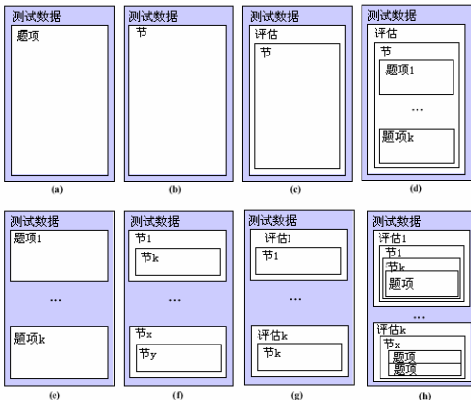
图4.1 主要的QTI数据结构
