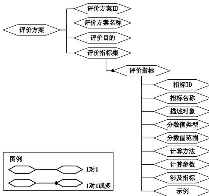
图2 在线课程评价方案信息模型
